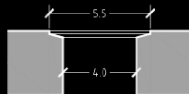
Sezione Scarico
