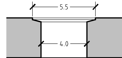
Sezione Scarico
