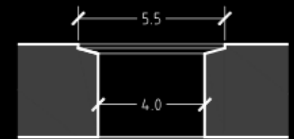
Sezione Scarico
